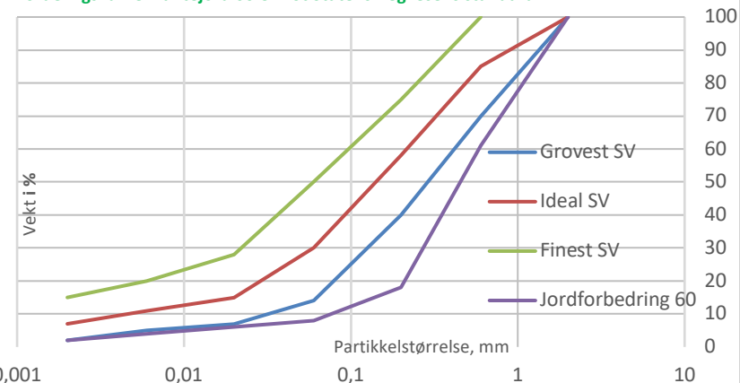
Kornfordelingskurve Plantejord 60 U mot Statens Vegvesens standard
