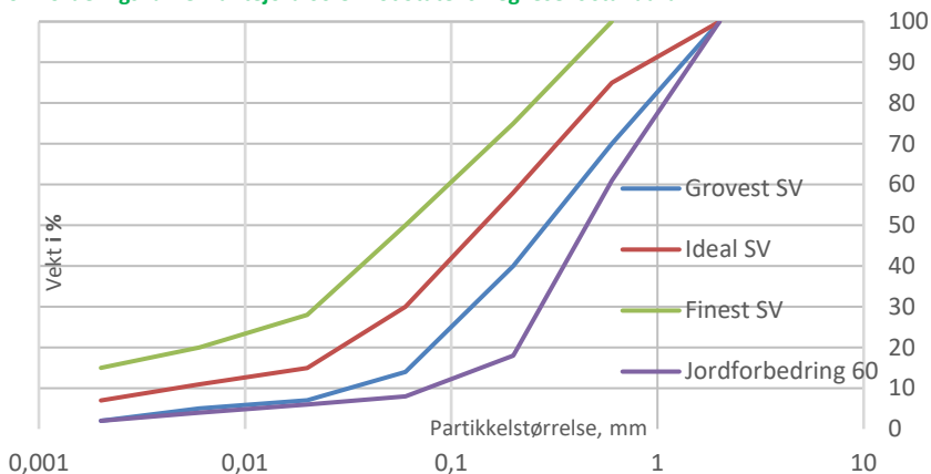
Kornfordelingskurve Plantejord 60 U mot Statens Vegvesens standard
